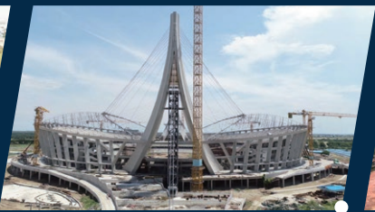
Morodok Techo National Stadium 國家體育場
